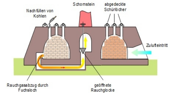
Schnitt durch den Ringofen
