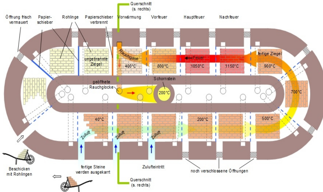
Hoffmannscher Ringofen der historischen Ziegelei Pape, Bevern
